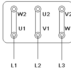
ANSCHLUß-CONEXIÓN Δ
