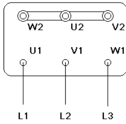
ANSCHLUß-CONEXIÓN Y
